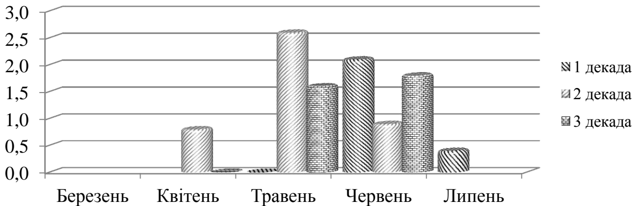
Рис. 1 Величина гідротермічного коефіцієнту за період від весняного відновлення вегетації пшениці м'якої озимої до воскової стиглості, 2013 р.
